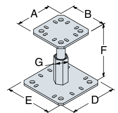
PPRC
