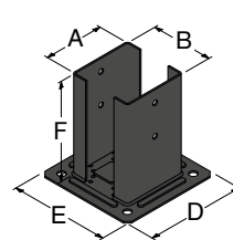
PPJNC70PB / PPJNC90PB
