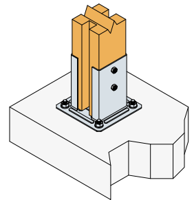
2 × Verbinderschraube Ø5×35 mm
